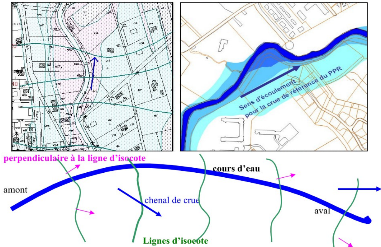
Sens d'écoulement des eaux : emprise de la ligne d'eau selon l'angle du bâtiment (exemples)
